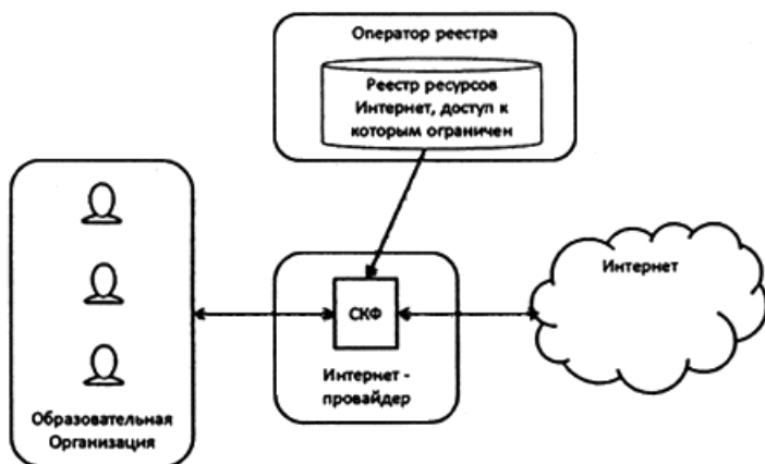
Рис.4. Схема работы контент-фильтрации при размещении у интернет-провайдера
