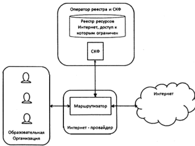
Рис.5. Схема работы контент-фильтрации при едином решении
